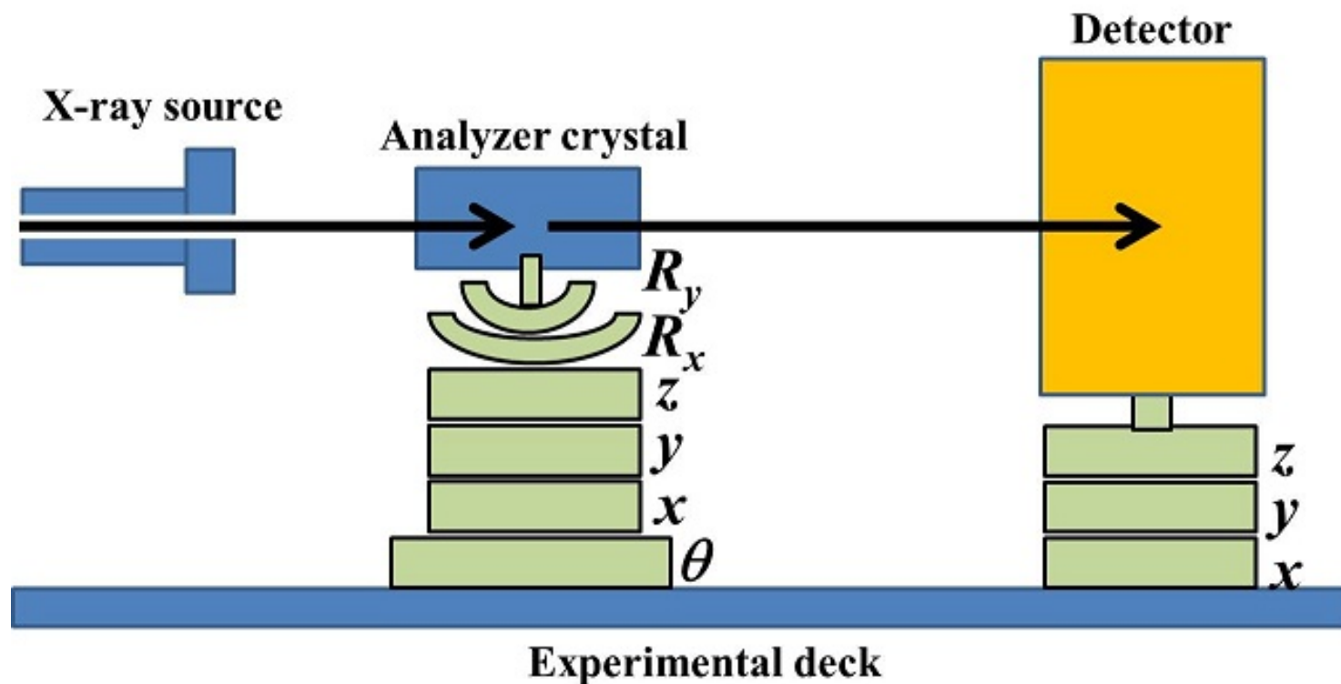
X線特性評価用実験装置模式図
