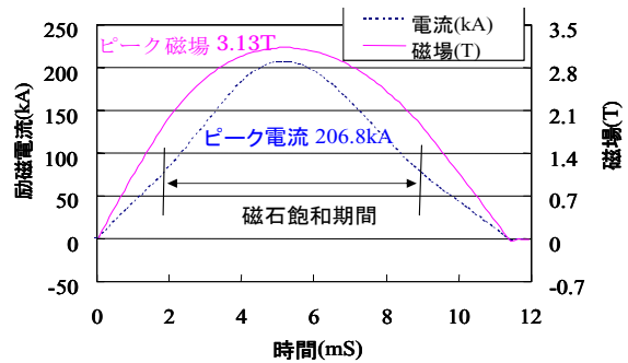
図3 偏向電磁石の励磁試験
