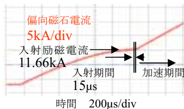
図8 入射用補助電源と既存電源を用いた偏向電磁石励磁試験
