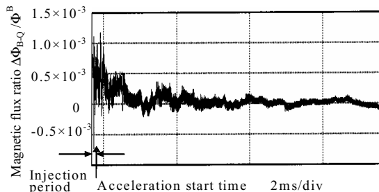
図10 偏向電磁石磁束と収束電磁石磁束のトラッキングシミュレーション
